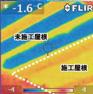
サーモグラフィー画像・冬
